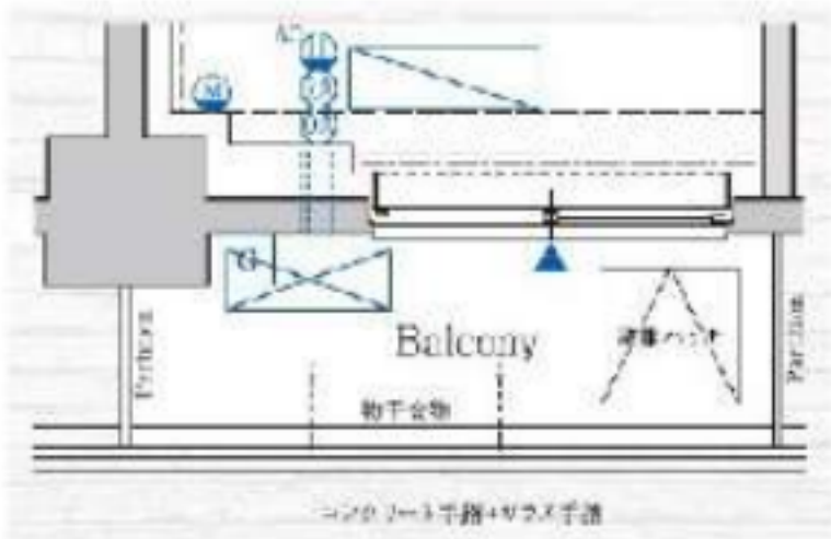
↑309号室 部分図
