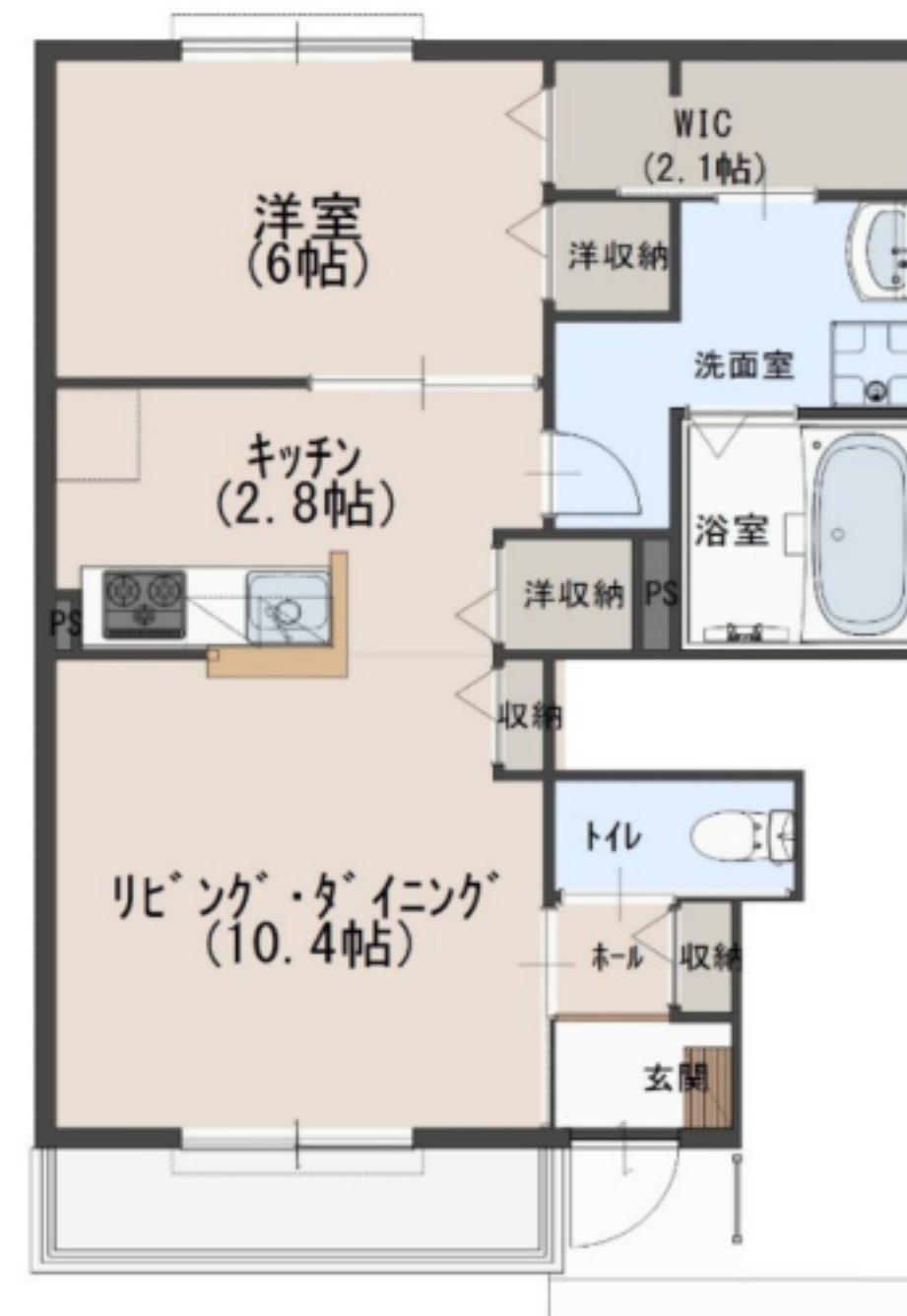
【間取】
