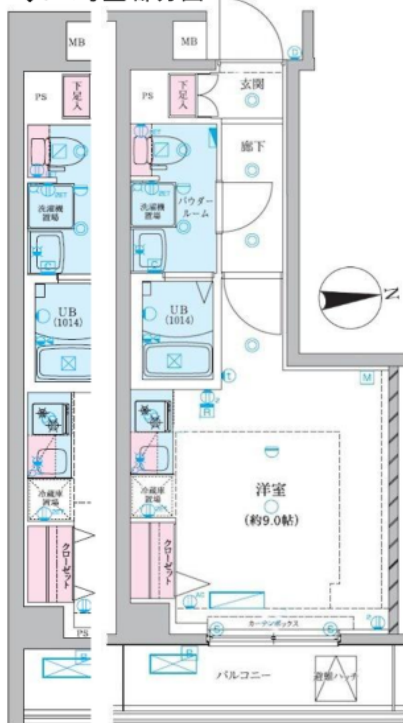
↓324号室 部分図
