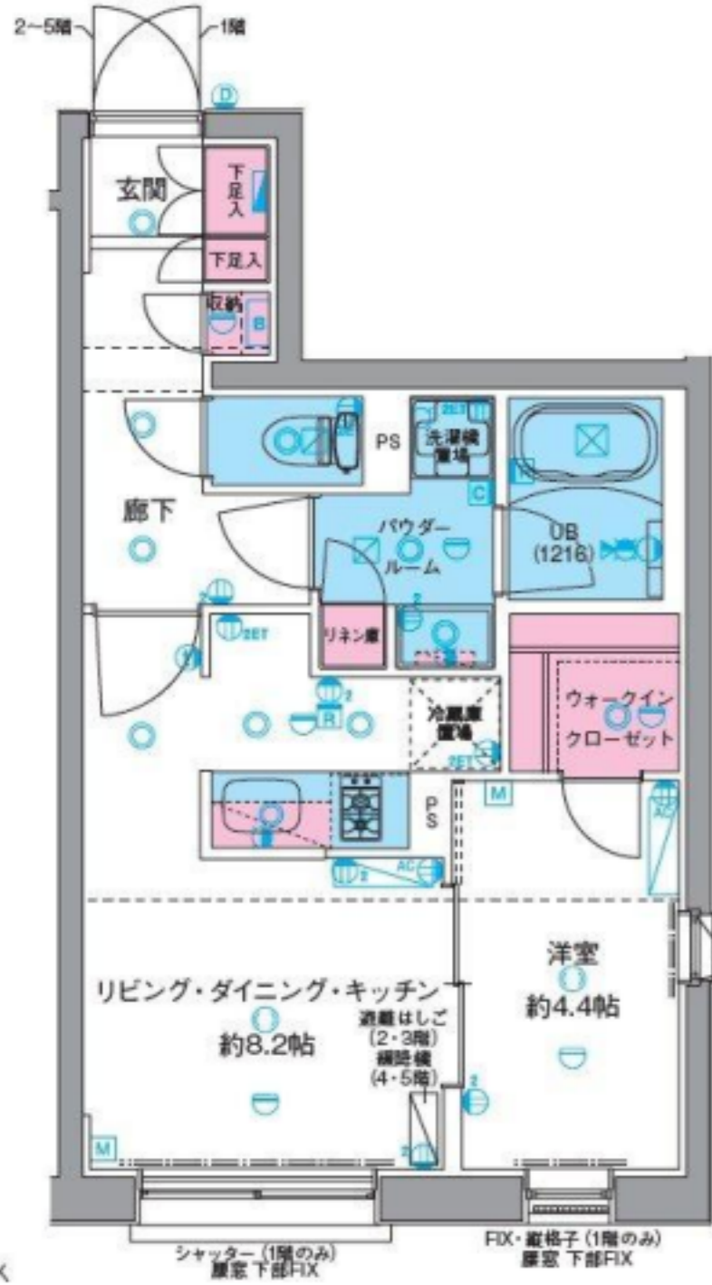
1階部分図
